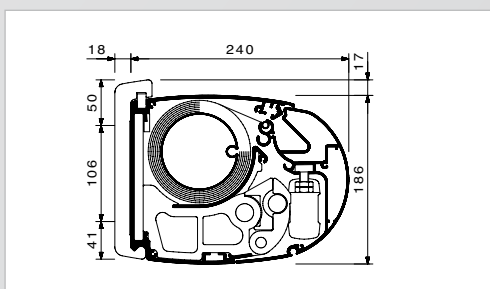
K500 Abmessungen
