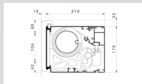
K450 Abmessungen
