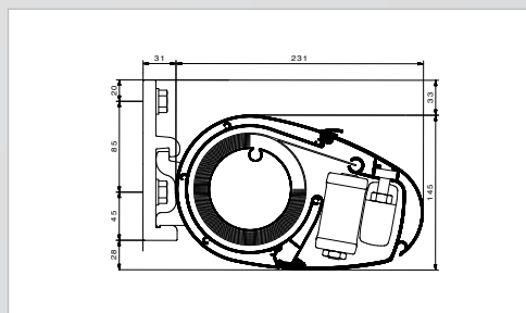
K200 Abmessungen
