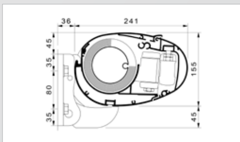
K350 Abmessungen
