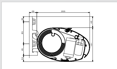
K100 Abmessungen
